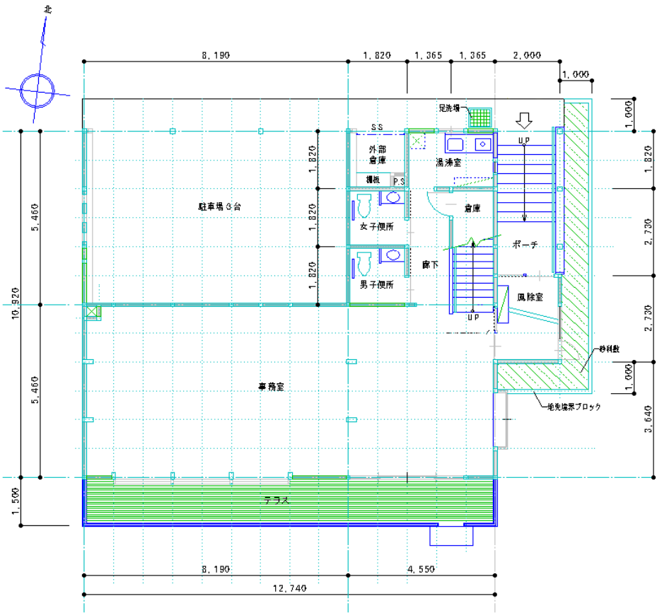
(1階)
